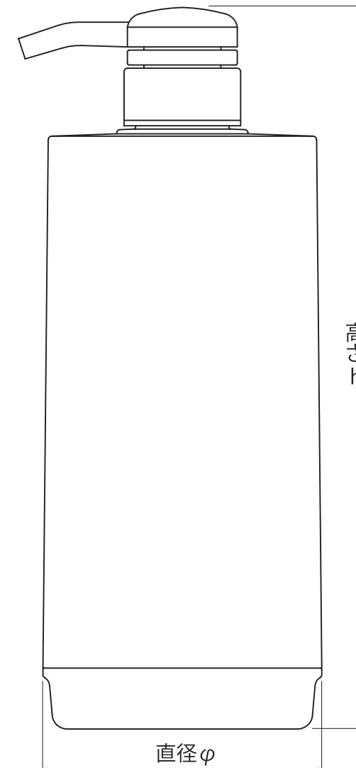
type:E 大容量ポンプ 600ml 吐出量：3ml
